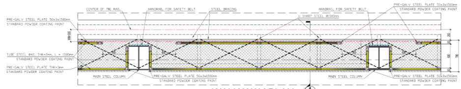
WALK WAY PLAN
